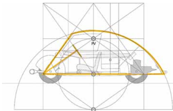
Voiture minimum, 1936, Le Corbusier. © FLC - ADAGP.
